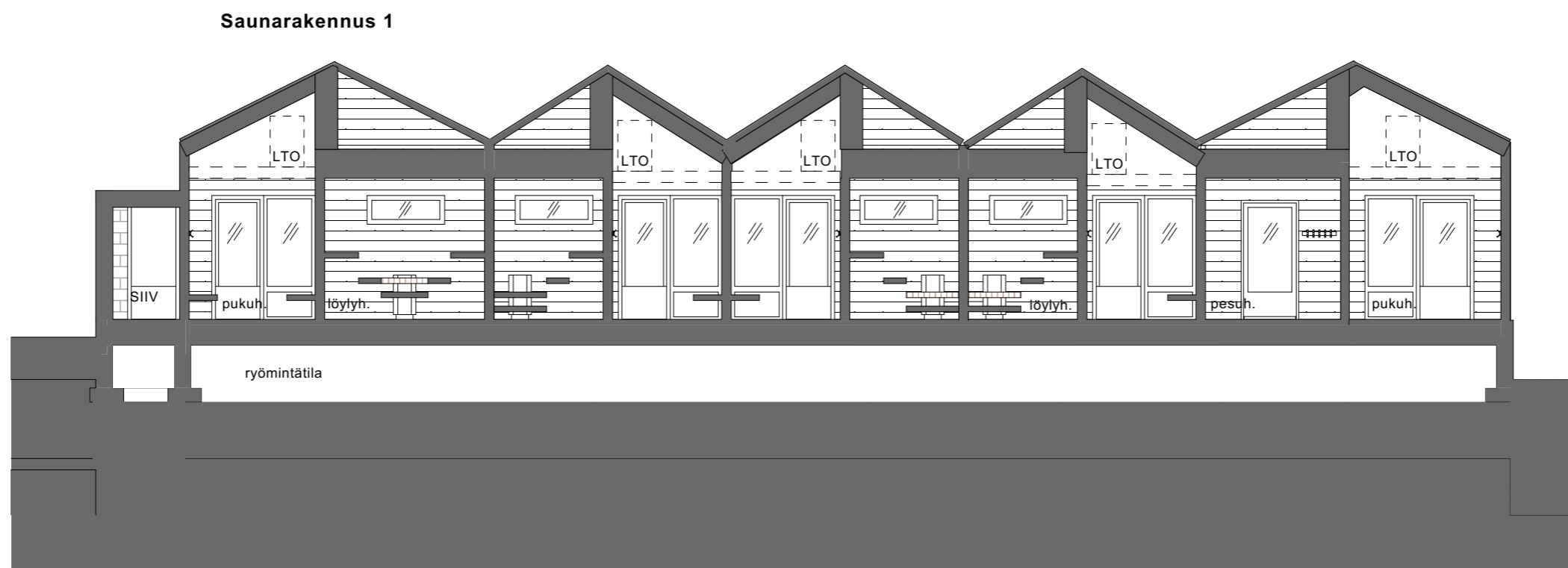
B-B Leikkaus
